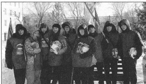
На открытии парка «Молодежный».
